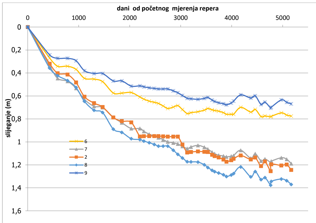
Slika 1. Prikaz konsolidacije repera broj 2, 6, 7, 8, 9 (profil 2). Horizontalna os prikazuje vrijeme u danima a vertikalna os prikazuje slijeganje u metrima. Vrijeme je prikazano u linearnom mjerilu. Početni datum mjerenja slijeganja je 24.11.2006.
